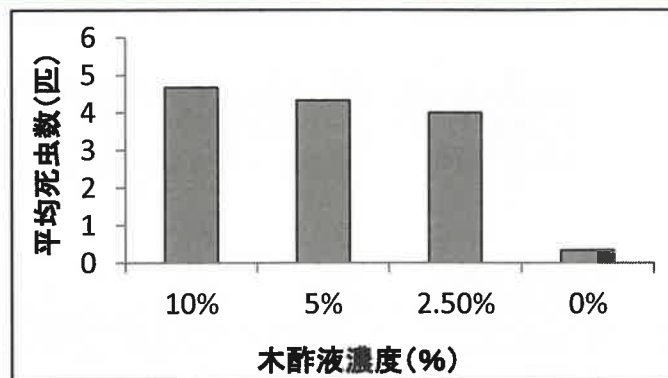
図1 木酢液を用いて行った殺ボウフラ試験の結果
