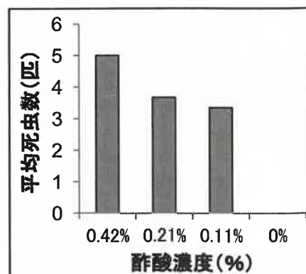
図3 酢酸を用いて行った殺ボウフラ試験の結果
