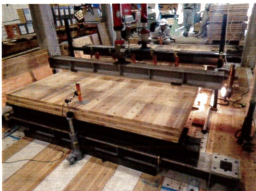
2.4m幅のCLTの曲げ試験
