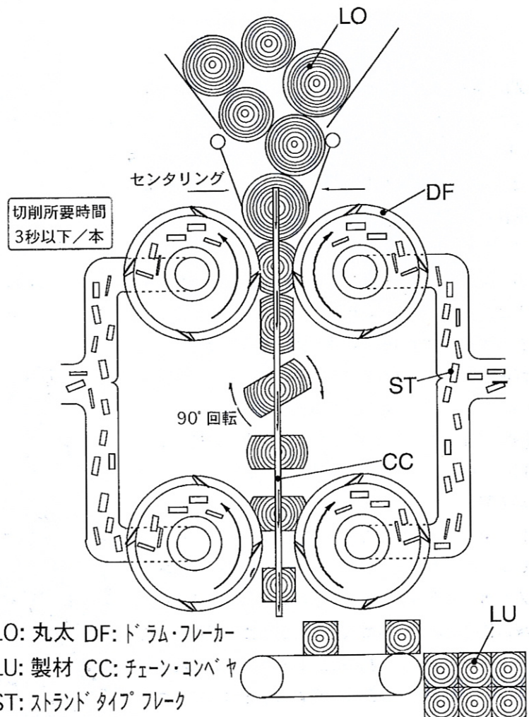
【図1】フレイキングミルの概念図
